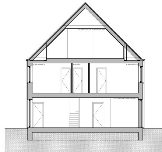
SNEDE
