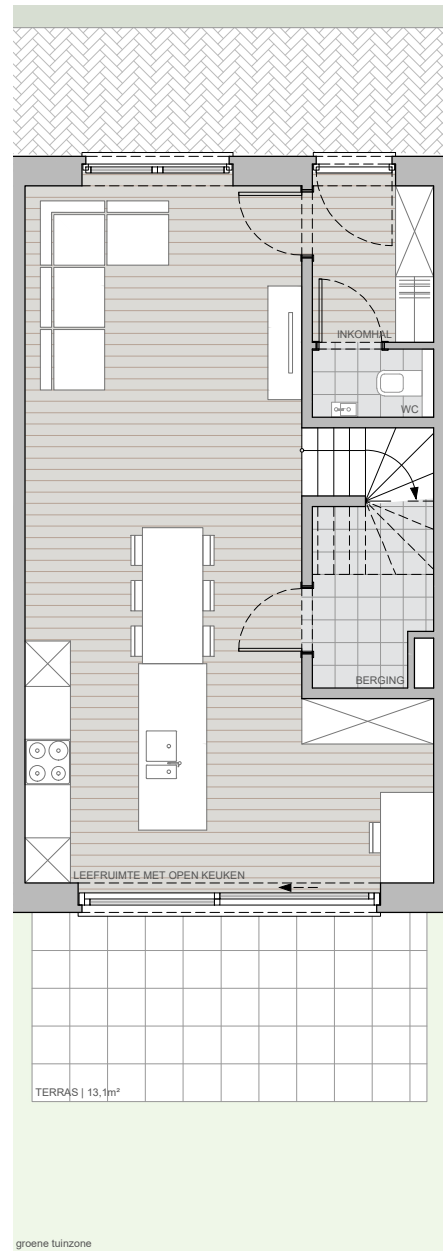
GRONDPLAN Niv. 0
