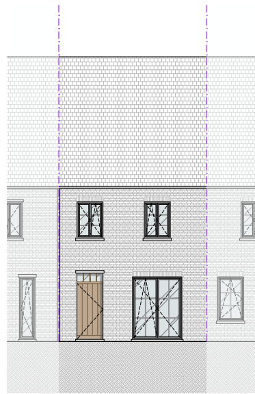
VOORGEVEL
